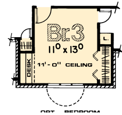
OPTIONAL BEDROOM
